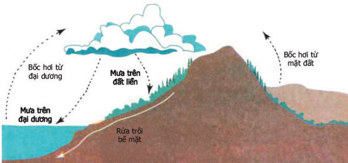
Hình 58.2. Chu trình nước trên Trái Đất
