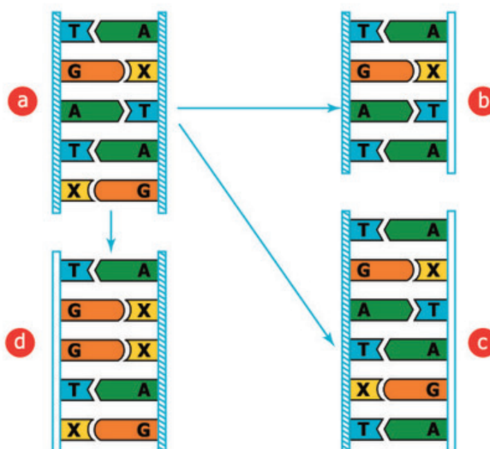
Hình 21.1. Một số dạng đột biến gen
