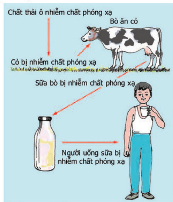
Hình 54.4. Sữa bò bị nhiễm chất phóng xạ
